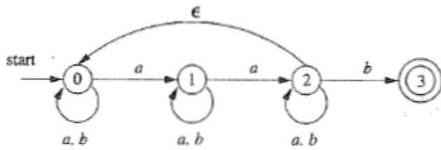
图 3-29 练习 3.6.3 的 NFA
