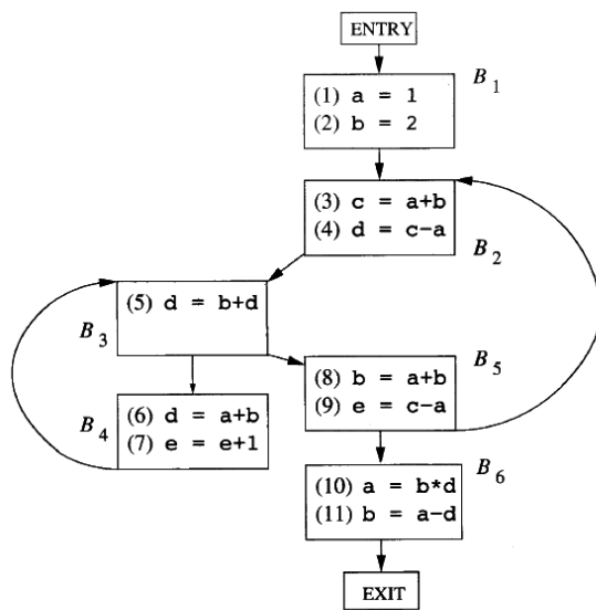
图 9-10 练习 9.1.1 的流图
