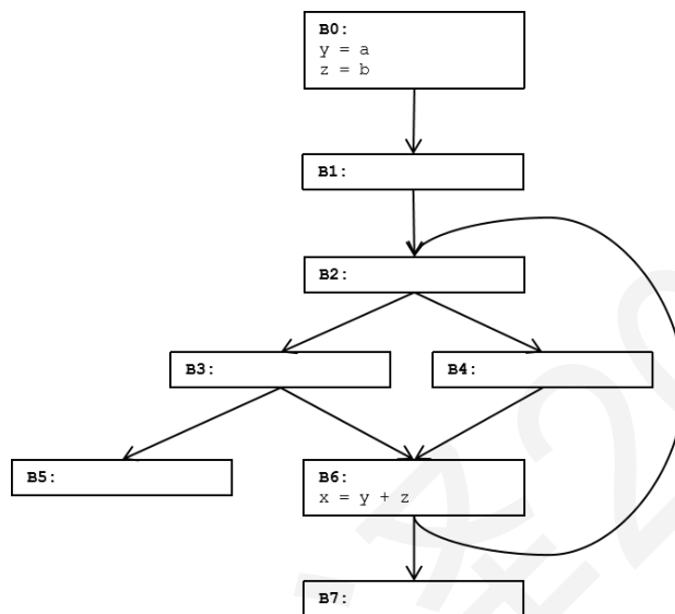
图 6.79 循环内部定义不能支配所有出口的示例
