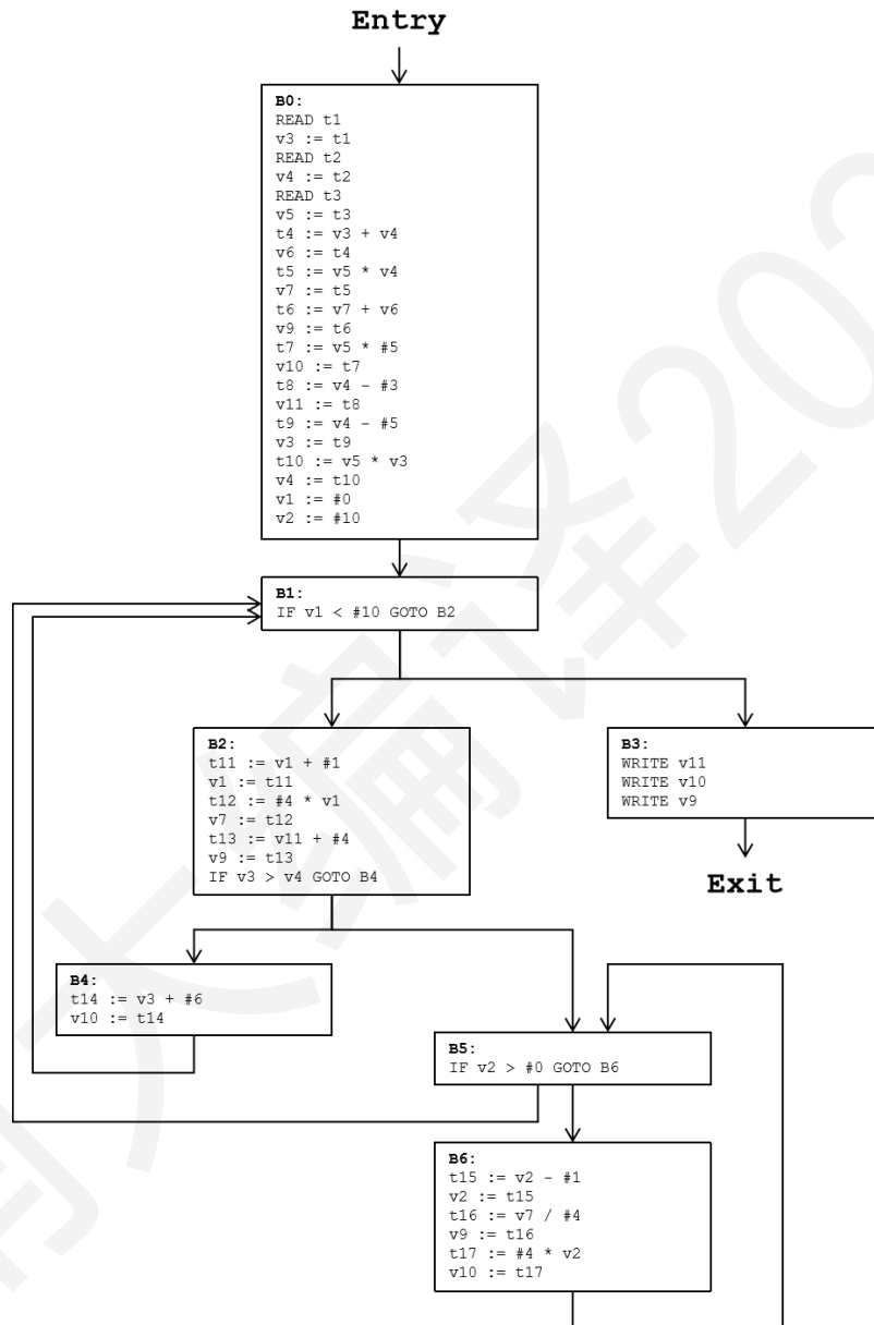
图 6.75 无用代码消除后的控制流图
