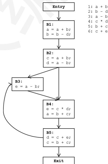
图 6.97 习题 6.3 的控制流图
