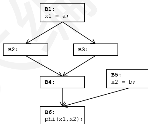
图 6.68 支配边界示例
