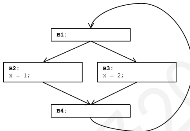
图 6.77 循环内部存在两条赋值语句示例
