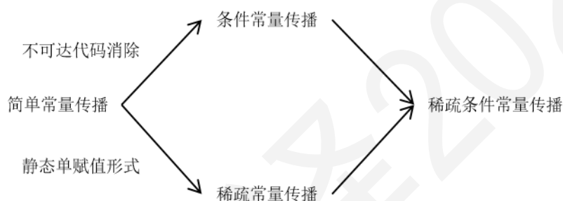
图 6.57 三种常量传播框架
