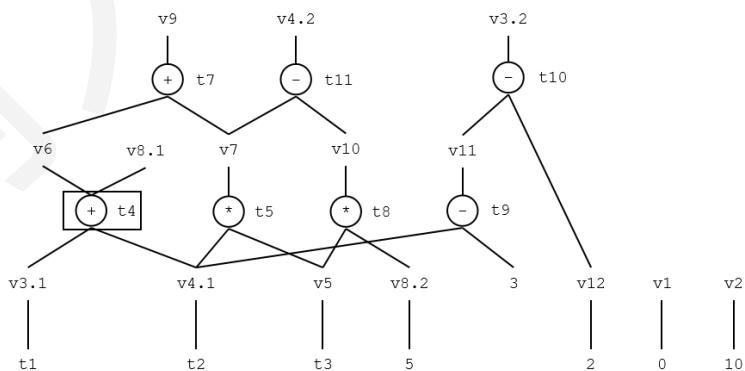
图 6.46 公共子表达式消除
