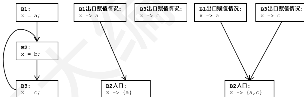
图 6.20 状态合并
