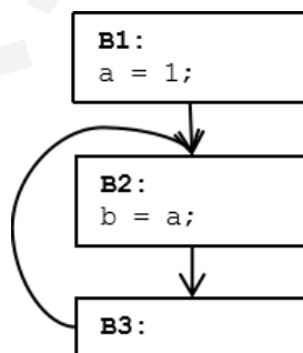
图 6.55 初始化示例
