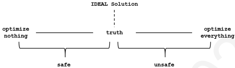
图 6.12 优化结果
