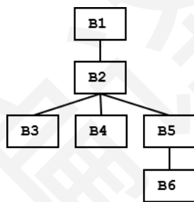
图 6.89 支配树
