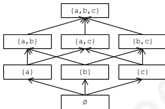
图 6.4 P(A) 上的偏序关系 \subseteq 的哈斯图
