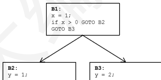
图 6.76 可达代码示例
