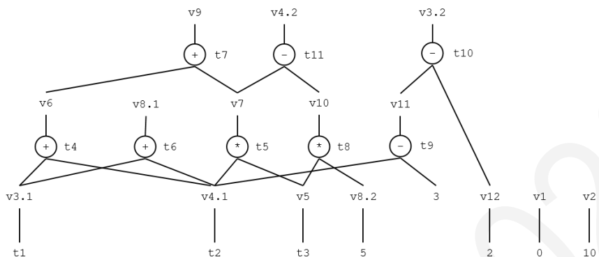
图 6.44 从中间代码生成的有向无环图
