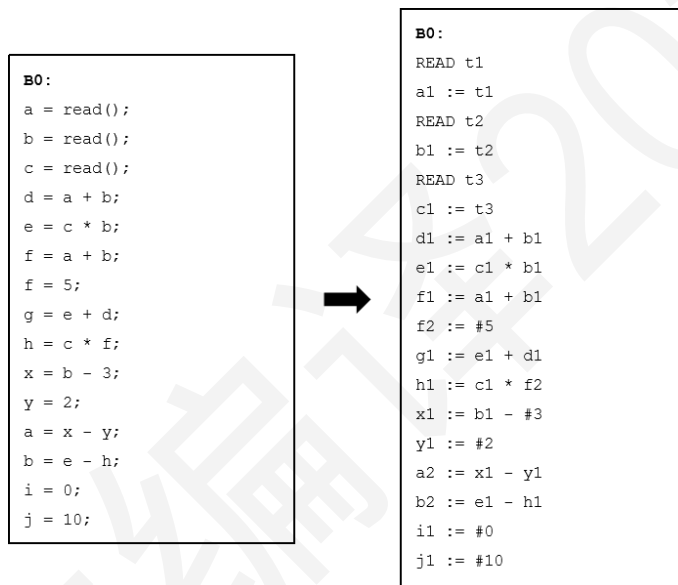
图 6.59 SSA form 中间代码
