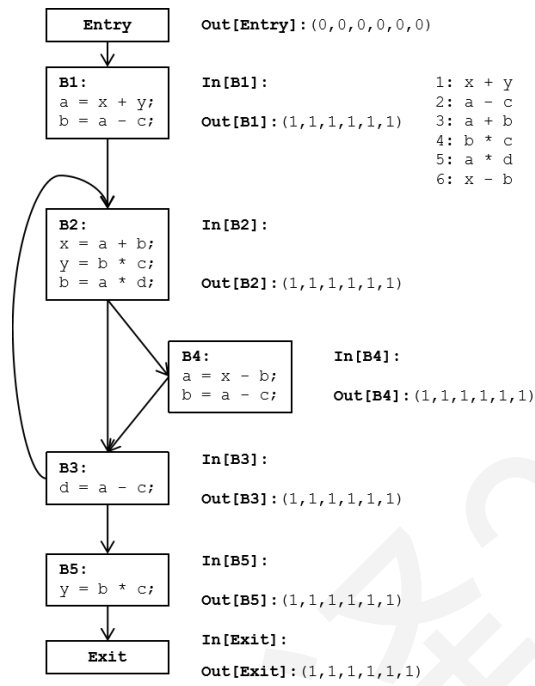
图 6.31 可用表达式模式初始化
