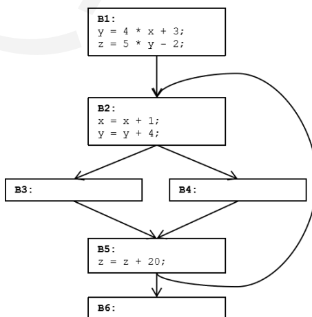
图 6.90 强度削减结果
