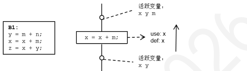
图 6.39 程序状态变化
