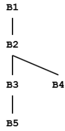
图 6.62 支配树
