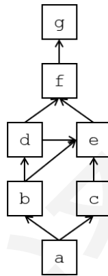
图 6.95 习题 6.1 的哈斯图
