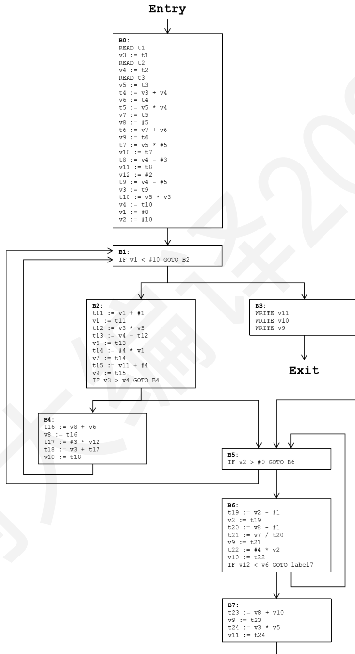
图 6.54 控制流程图
