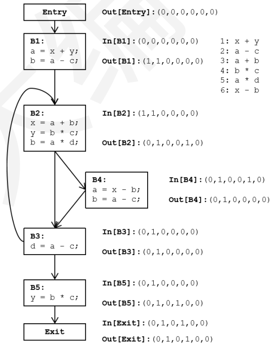
图 6.32 第一次迭代结果
